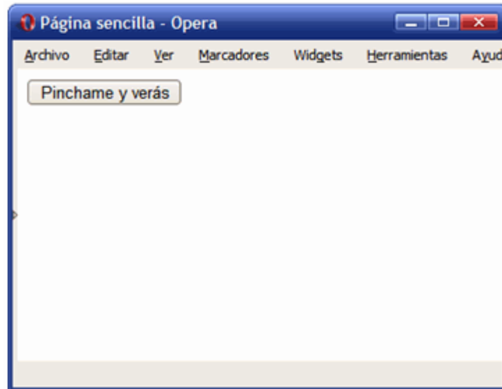
Figura 6.1. Página HTML
